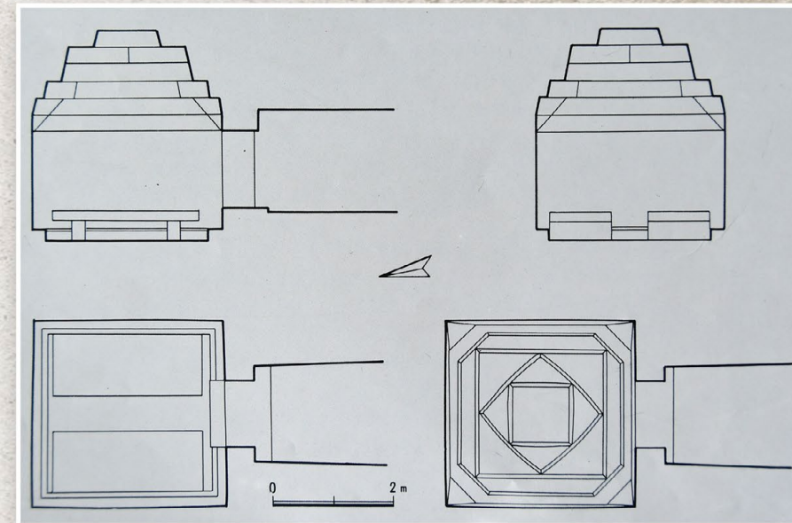
Эскиз погребальной камеры.
