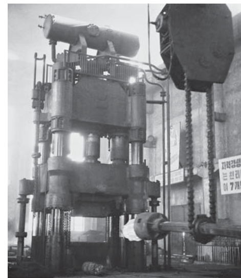
Трактора «Чхоллима», произведенные на Киянском (сегодня Кымсонский) тракторном заводе. (↑) Изготовленный на Рёнсонском машиностроительном заводе пресс с давлением 3000 тонн. (←)
